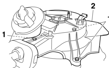
1. Болты 2. Крышка ручного стартера/махового колеса с магнитами
