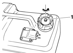
1.Винт вентиляционного отверстия
