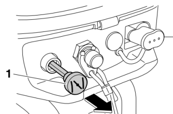
1. Ручка обратного клапана
