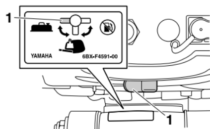
1.Положение, соответствующее съемному топливному баку
