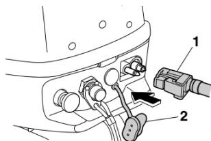
1.Топливный шланг 2.Крышка соединителя подачи топлива
