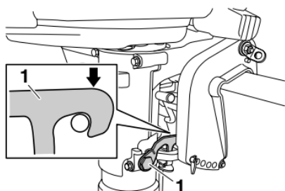
1. Фиксатор наклона
