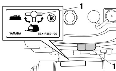
1. Закрытое положение
