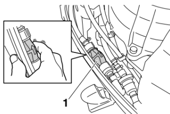
1.Насос подкачки
