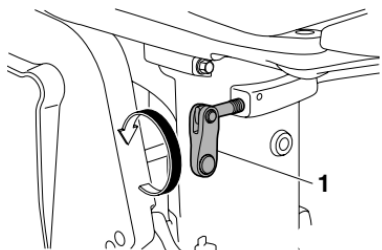
1. Фрикционный регулятор рулевого управления
