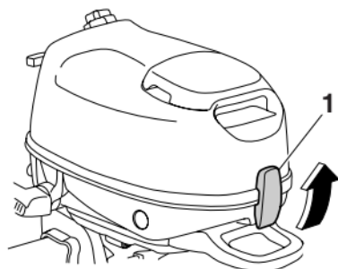
1. Рычаг замка верхней части кожуха
