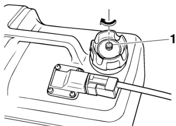
1. Винт вентиляционного отверстия
