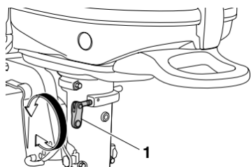
1. Фрикционный регулятор рулевого управления
