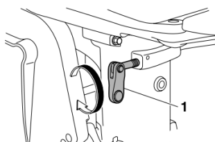
1. Фрикционный регулятор рулевого управления
