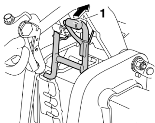
1. Упор для поддержания мотора в полностью наклоненном положении
