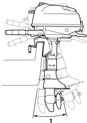
1. Рабочий угол триммера
