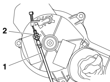
1. Трос системы защиты двигателя от случайного запуска 2. Гайка
