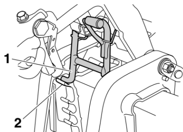
1. Упор для поддержания мотора в полностью наклоненном положении
